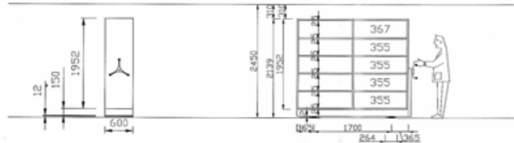
Разрез модул F
