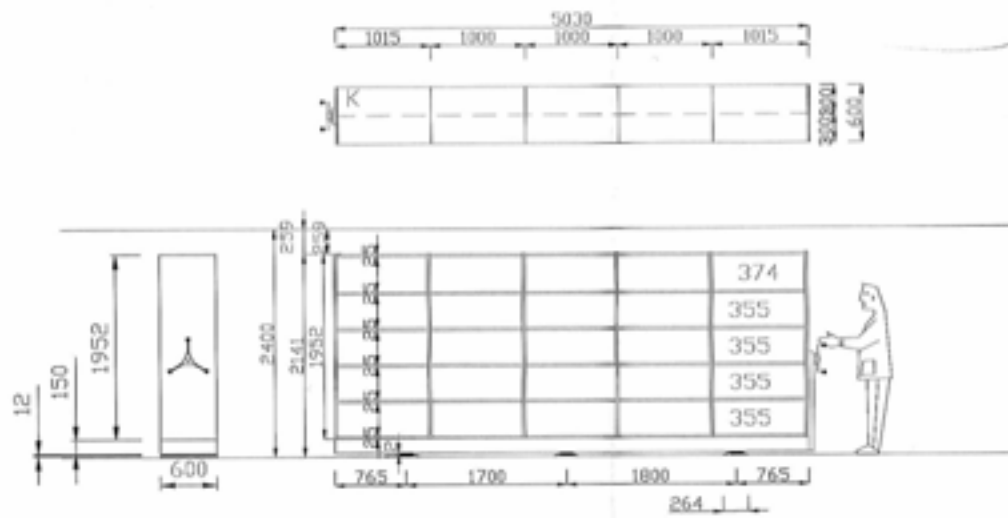
Разрез модул К
