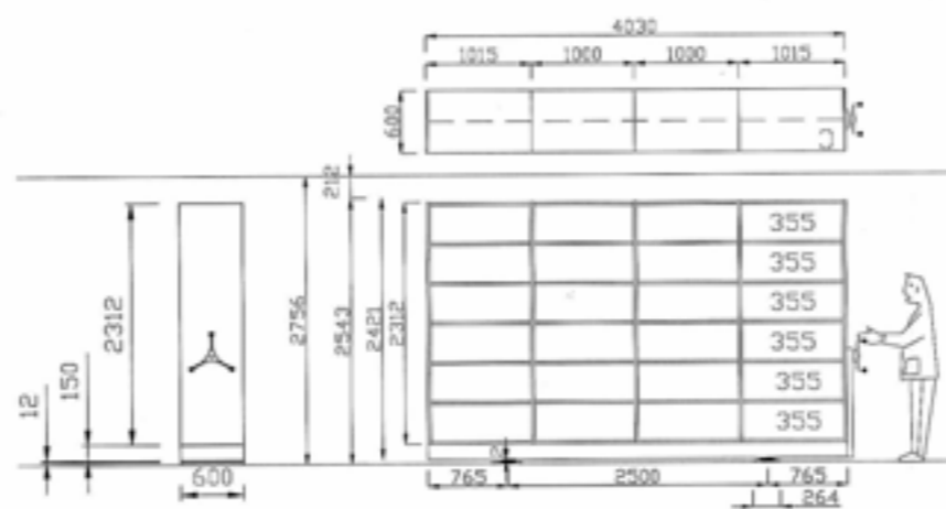
Разрез модул С
