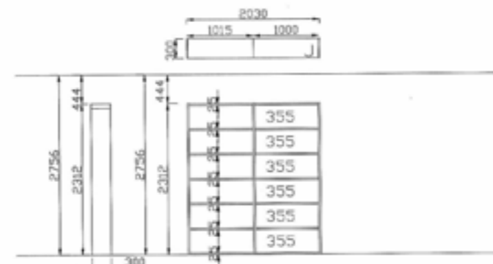
Разрез модул J
