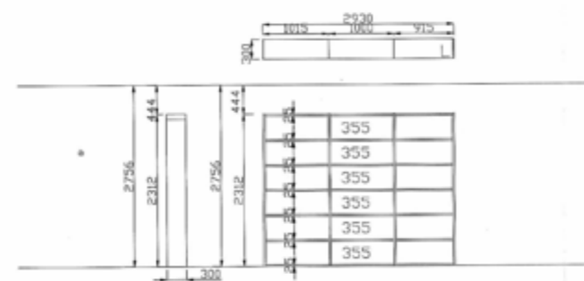
Разрез модул L
